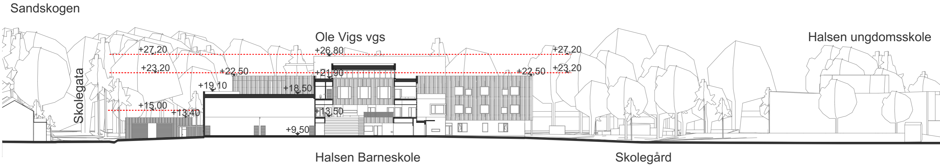
Snitt 1
