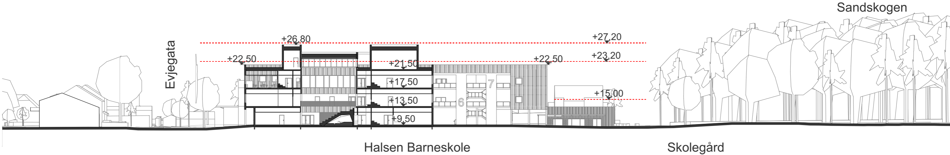
Snitt A
