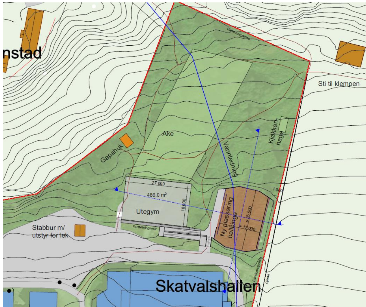
Figur 14 Illustrasjon av mulig løsning for uteareal bak Skatvalshallen (S.A.K) Endelig løsning må ta hensyn til innspill mottatt fra skolen og beskrevet i planbeskrivelsen. Rampe bør ha nedre adkomst fra vestlig retning da de fleste brukerne kommer fra vest, akebakke må ivaretas bedre og areal til ny ballbinge og utegym bør derfor samles og trekkes østover. Kjøreadkomst til flater må sikre for rasjonell drift av området. Det er ønskelig med isbane på vinterstid og denne bør kunne brøytes og islegges fra maskinelt utstyr.
