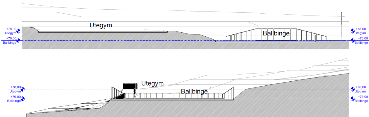
Figur 16 Terrangsnitt av mulig opparbeidelse av uteareal nord for Skatvalshallen (S.A.K) Illustrert løsning må bearbeides videre.
