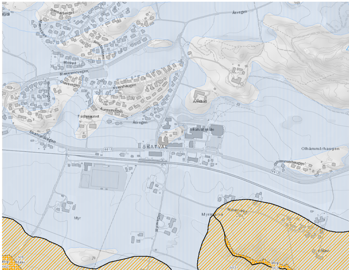
Figur 9 Blå skravur viser aktsomhet for marin leire, oransje skravur viser kvikkleiresoner. Kilde: NVE Atlas
