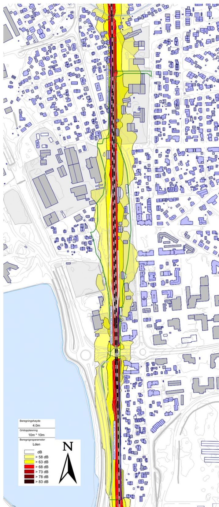
Figur 7 Utsnitt fra støykart X221 – Framtidig situasjon og togtyper – som viser områder med overskridelse av anbefalt grenseverdi i 1,5 m høyde inkl. foreslåtte langsgående støyskjermer.
