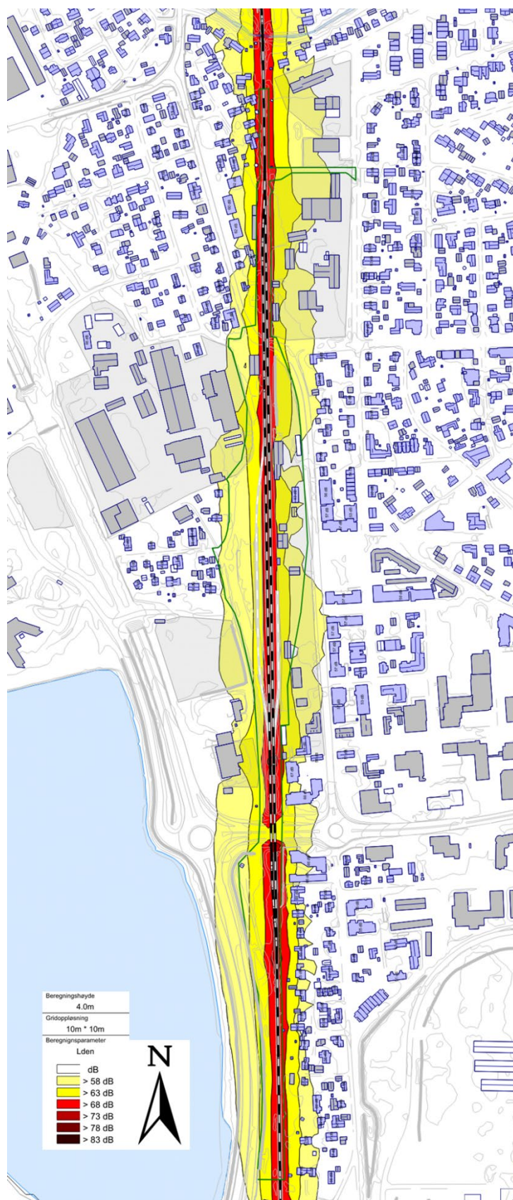
Figur 5 Utsnitt fra støykart X141 – Framtidig situasjon og togtyper – med utbredelse av gul og rød sone 4 m.o.t. iht. T-1442.
