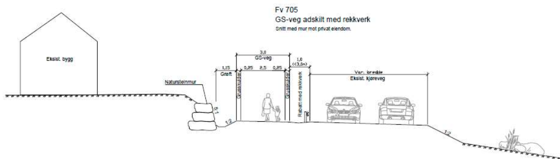
Figur 15 Normalprofil gang- og sykkelveg med rekkverk mellom gang-/sykkelveg og fv. 705. profilet viser natursteinmur mot bebyggelse
