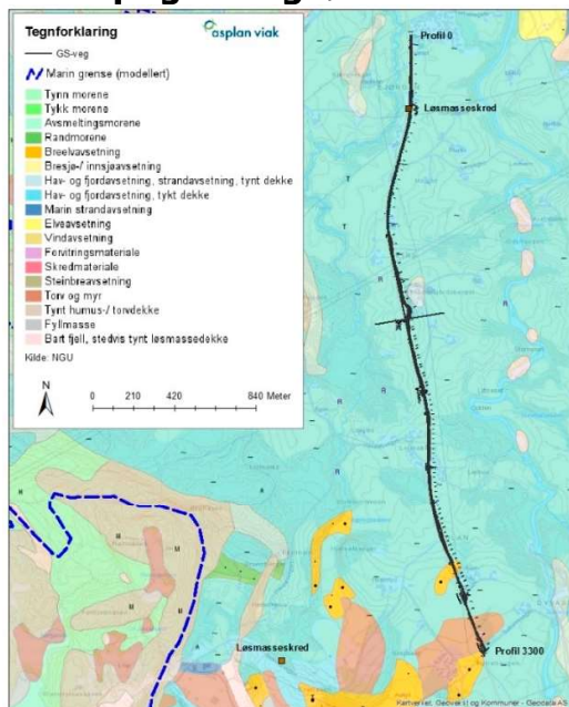
Figur 9 Løsmassekart for prosjektet (kilde: NGU). Trase for ny GS-veg er inntegnet med sort strek.
