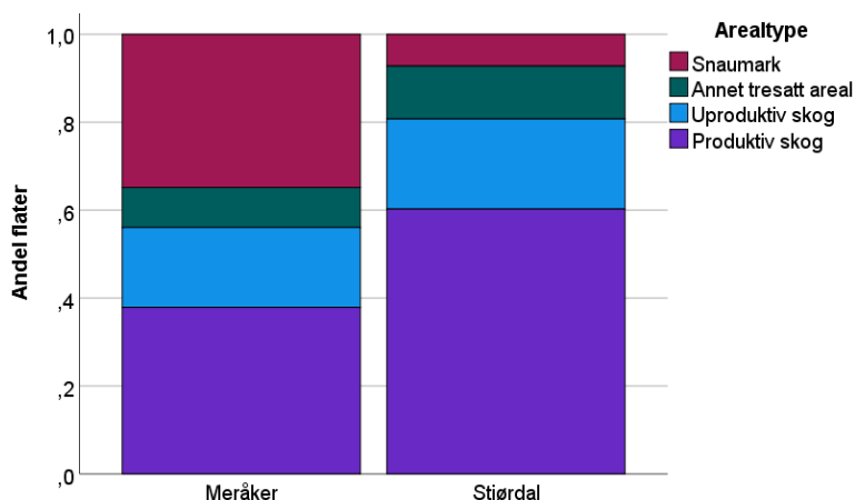
Figur 3.6.1. Andelen prøveflater på ulike arealtyper i skogsmark i Meråker og Stjørdal i perioden 2015–2019. Totalt antall prøveflater var 66 i Meråker og 83 i Stjørdal. Annet tresatt areal og snaumark er i hovedsak myr med og uten tresetting. Kilde: Landsskogtakseringen.
