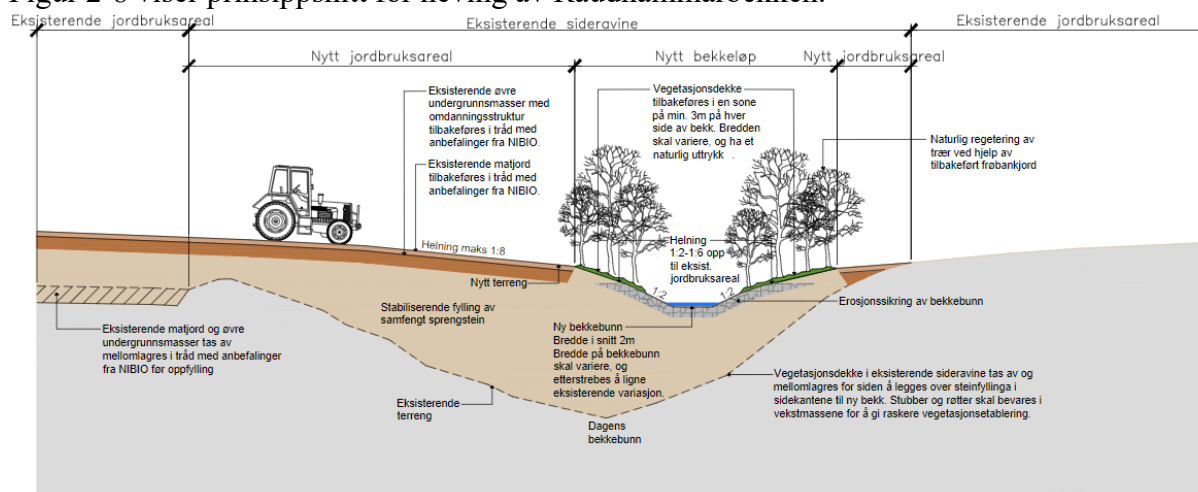
Figur 2-8 Prinsippsnitt heving av Raudhåmmårbekken etter stabiliserende tiltak.
