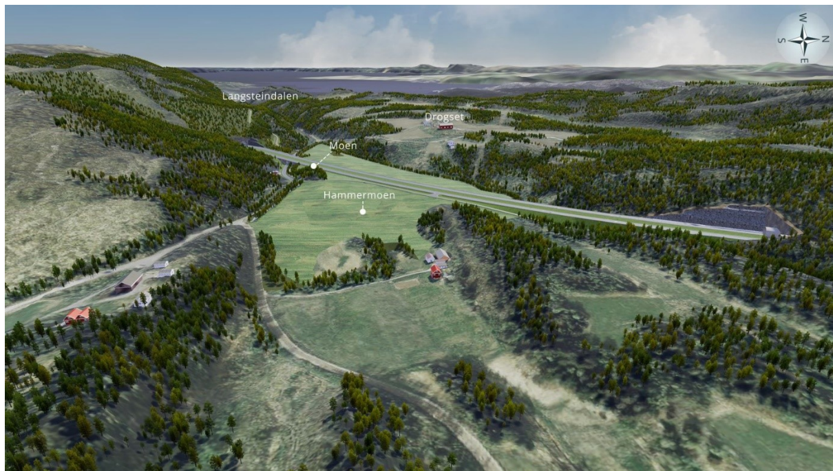
Figur 2-4 Veglinja krysser Langsteindalen. Retning Stjørdal mot venstre, retning Levanger mot høyre. Trondheimsfjorden i bakgrunnen
