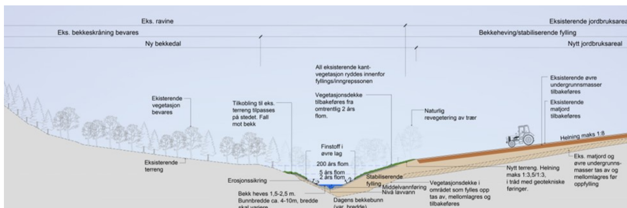
Figur 2-7 Prinsippsnitt øst: heving av Vollselva 1,5-2,5 m., inkludert stabilisering av nordlige sidekant i ravinen. Illustrasjon: Selberg Arkitekter 2020.
