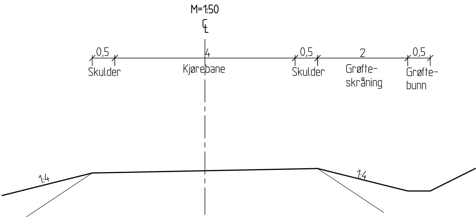
Normalprofil Adkomstveg rasteplass Linje 61300
