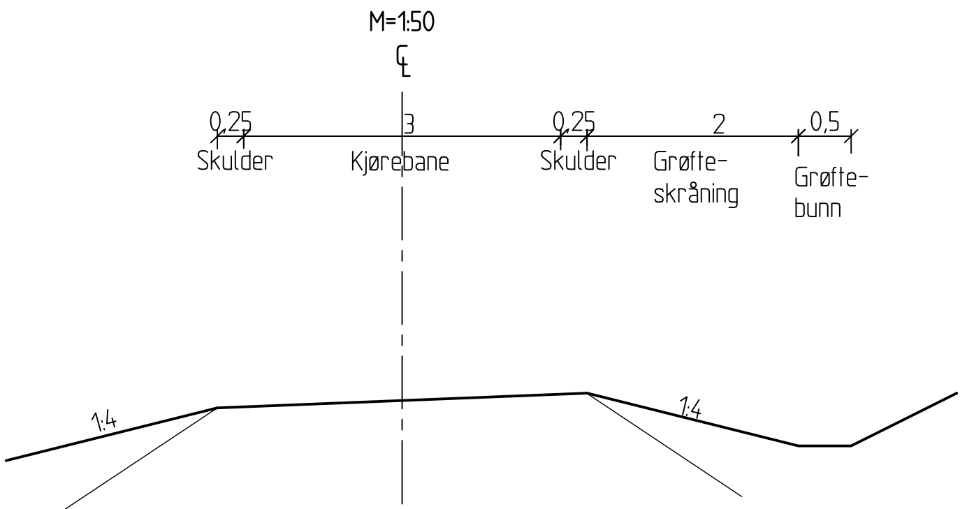
Normalprofil Gang- og sykkelveg
