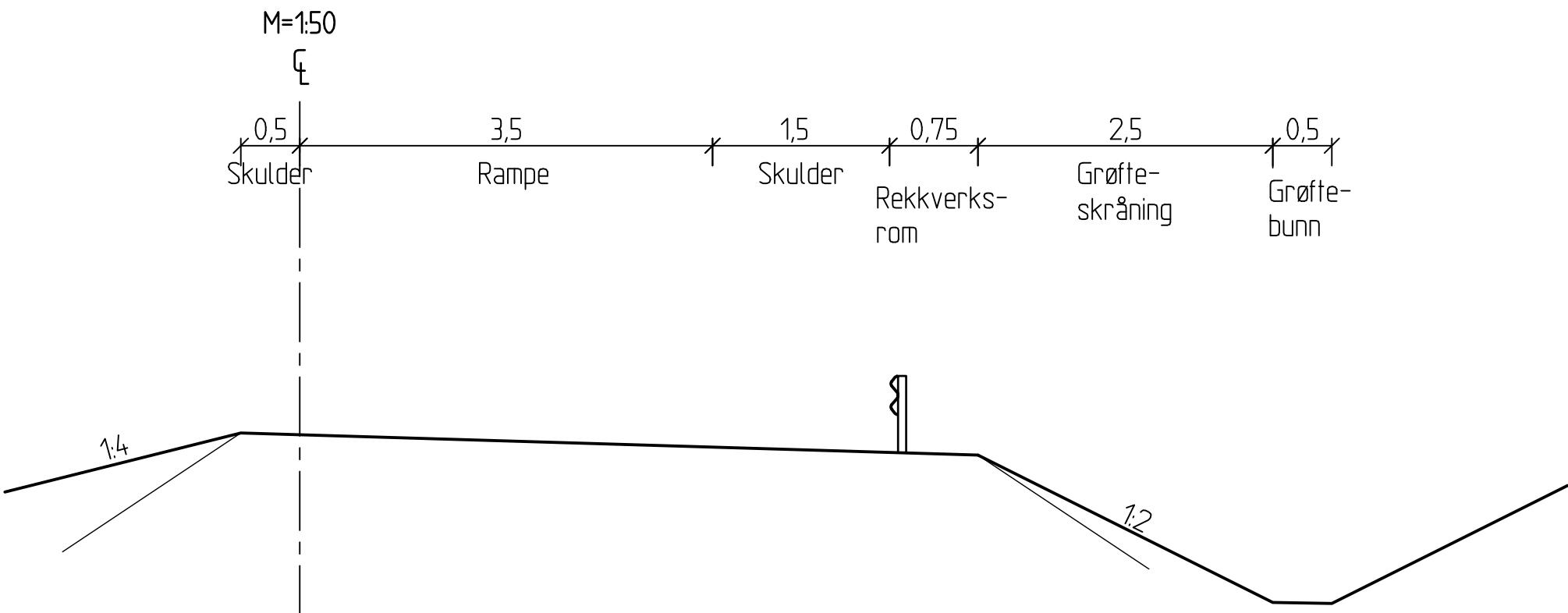
Normalprofil Rampe m/rekkverk
