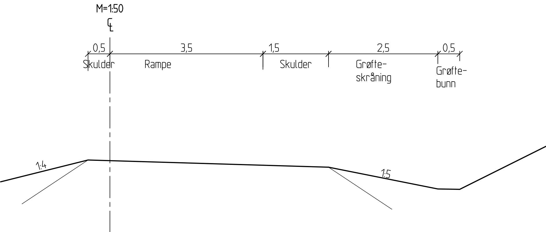
Normalprofil Rampe
