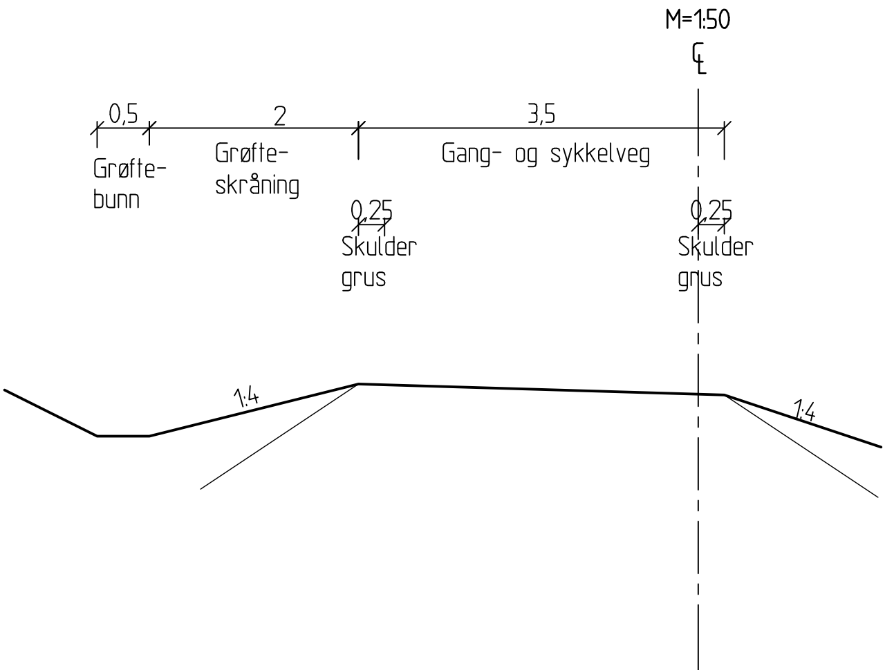
Normalprofil Rampe
