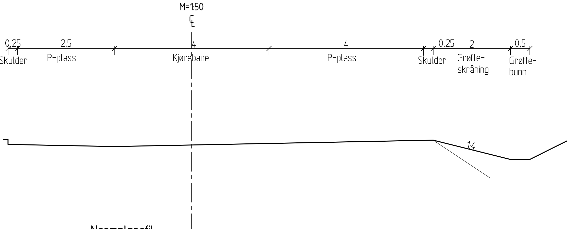
Normalprofil Rampe m/rekkverk
