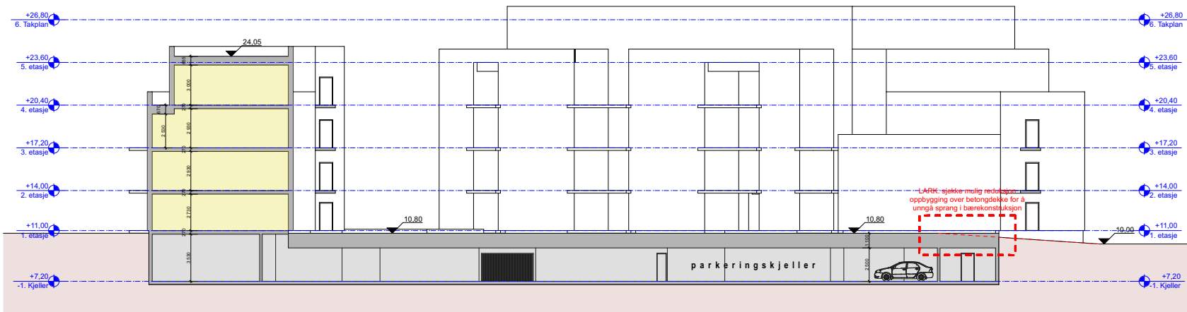
1:400 Snitt 1
