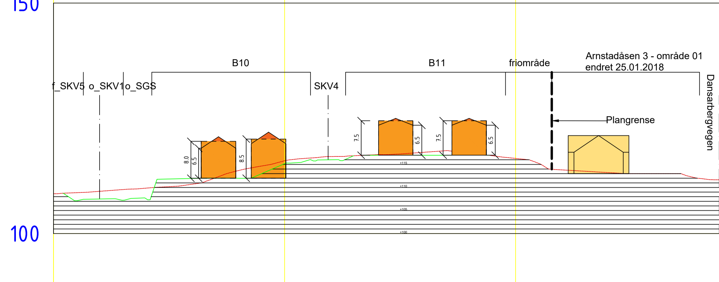
150 Snitt A
