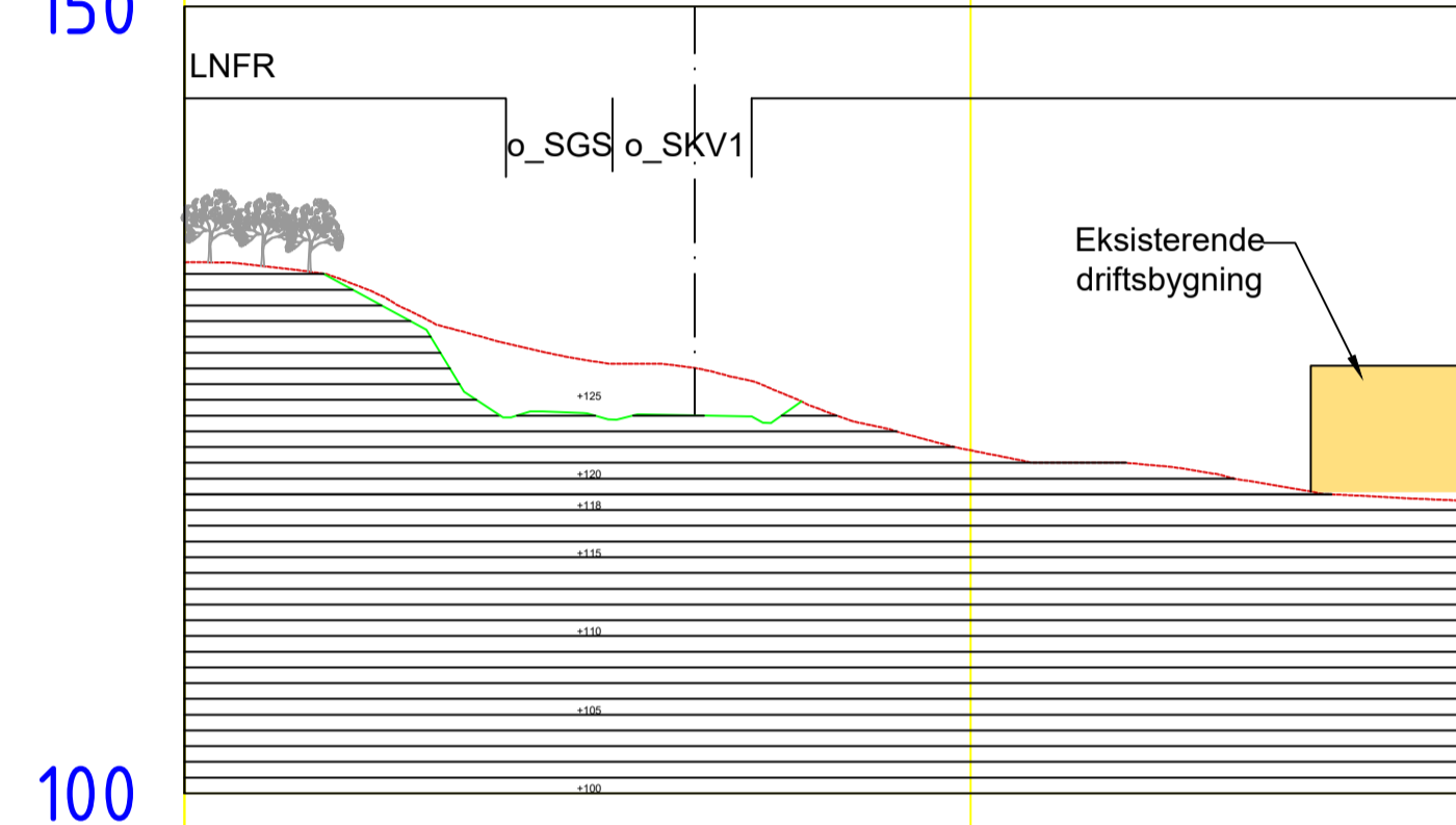
150 Snitt D
