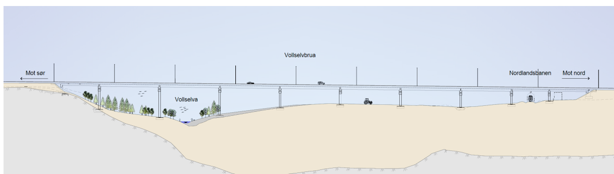
Figur 22: Bru over Vollselva og jernbanen i Vollsdalen [4].
