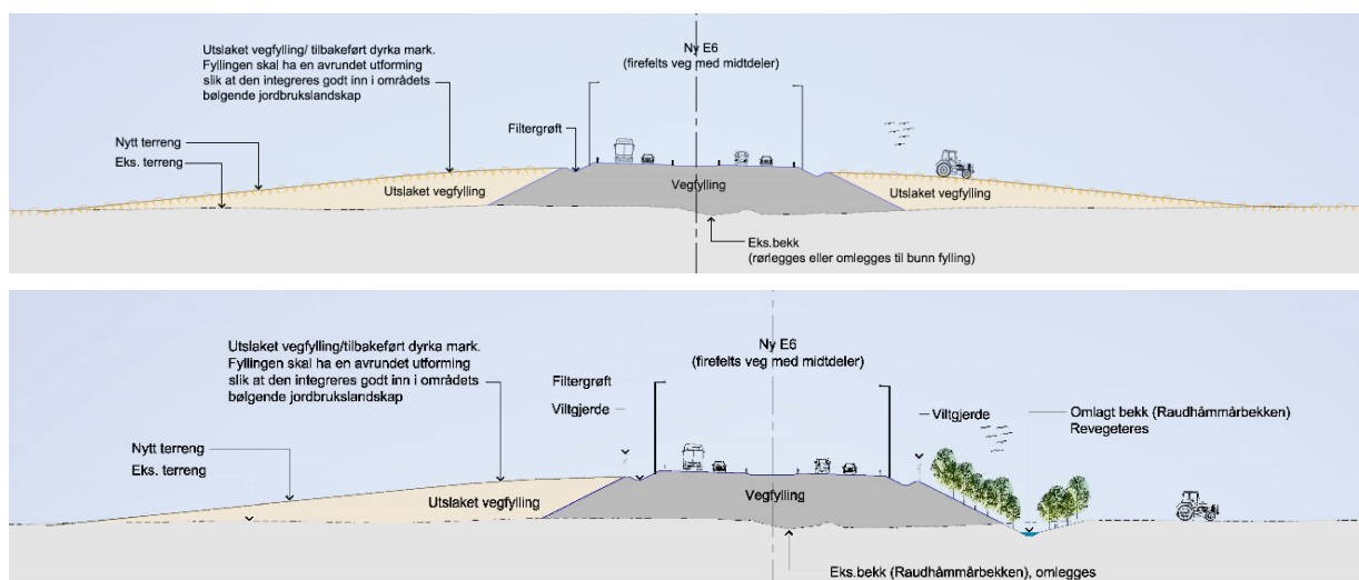
Figur 23: Prinsipp benyttet gjennom jordbrukslandskapet ved Volla, sør for Vollsдалen, vist i øverste illustrasjon. Nederst vises prinsipp benyttet mellom jernbanen og tunnelportalen ved Holan.
