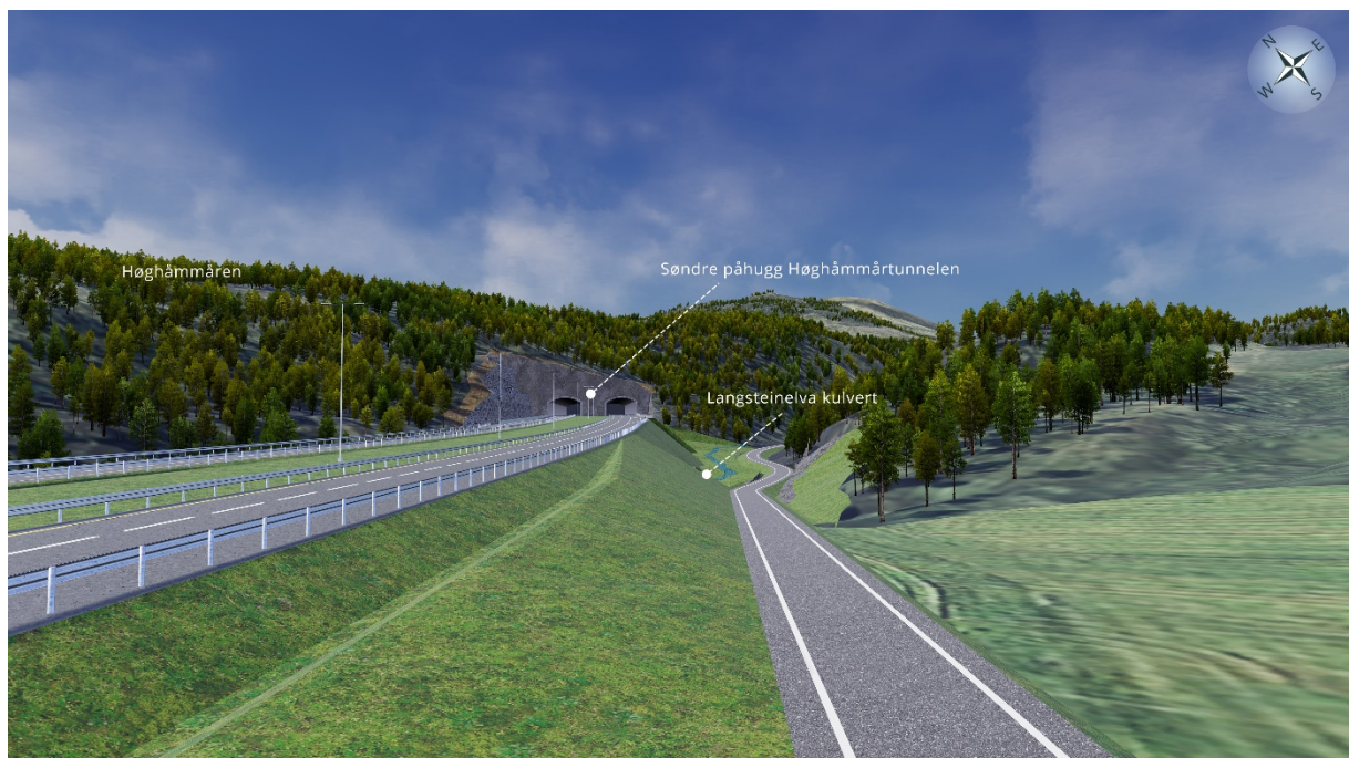
Figur 58: Bakkeperspektiv sett fra sørvest mot nordøst og tunnelpåhugget til Høghåmmårtunnelen. Tunnelportalene, og ikke minst skjæringene, vil være godt synlig i landskapet, og bryter med eksisterende landskapskarakter i delområdene. Synligheten til påhugget forsterkes av at vegen samtidig ligger på en relativ høy fylling i forkant av tunnelmunningen. Langsteinelva skal i ny situasjon krysse under E6 i en kulvert. Det går en atkomstveg parallelt med E6 i ny situasjon.
