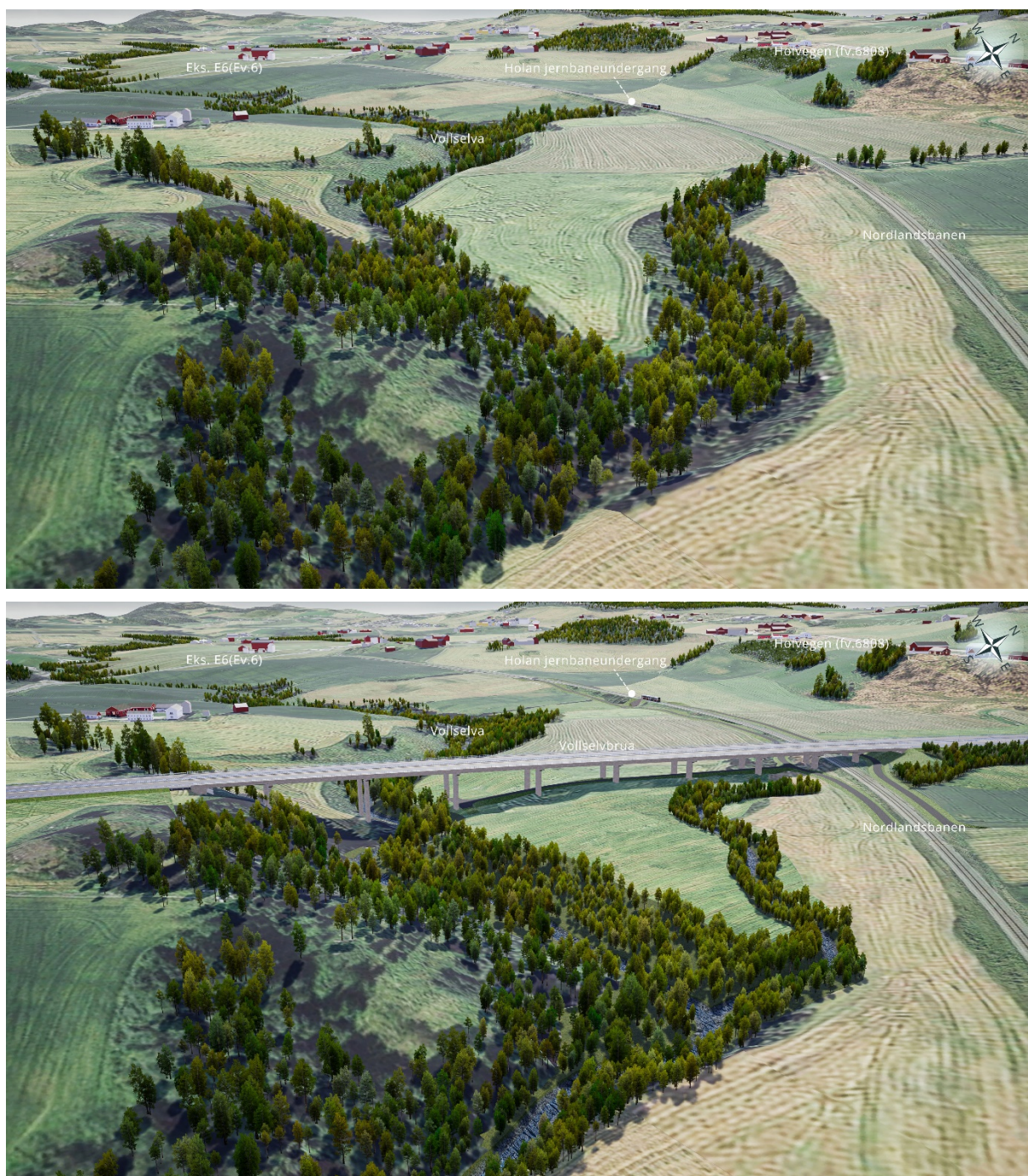
Figur 28: 3D-luftperspektiv av dagens og framtidig situasjon med Vollselvbrua over Vollsdalen, sett fra øst mot vest. Det må gjøres geoteknisk stabilisering av Vollsdalen ved oppfylling av masser i sideraviner, samt heving med erosjonssikring av Vollselva. Vollsdalen vil fortsatt oppleves som et viktig strukturelt og gjenkjennbart landskapselement i området, men med en noe «strammere» overgang mot omliggende jordbrukslandskap.
