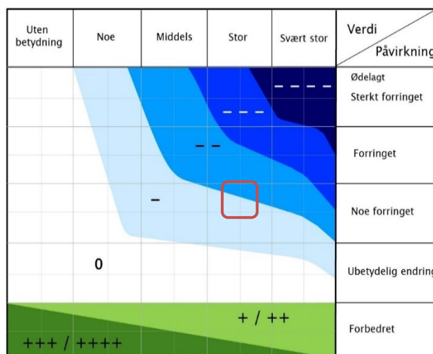
Figur 36: Konsekvens [2, p. 119], delområde 1, Voll-Holan.
