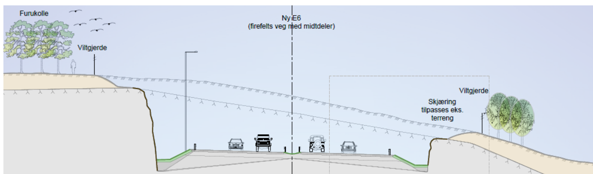
Figur 21: Prinsippsnitt for skjæring ved Vollan [4].
