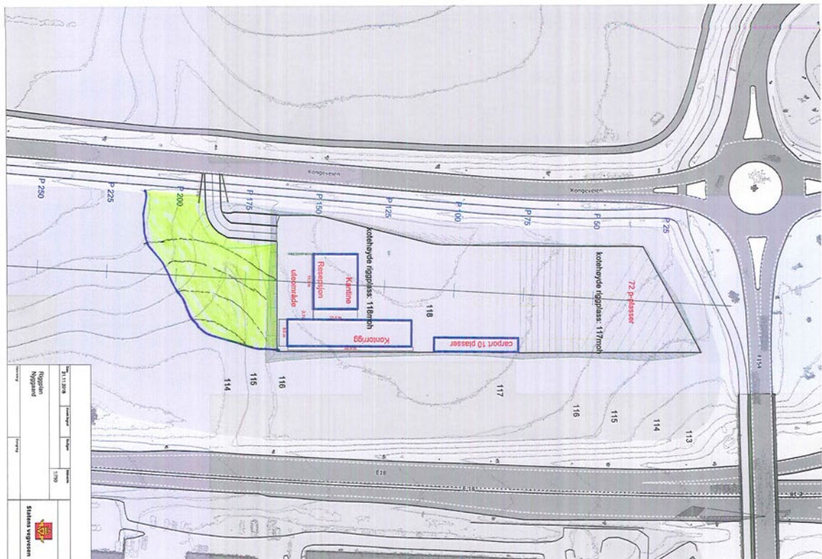
Figur 12 Midlertidig oppfylling av terreng sør for riggområde med masser av ploglaget fra riggområdet (Legg merke til forskjellen på gamle og nye koter på oppfyllingsområdet).
