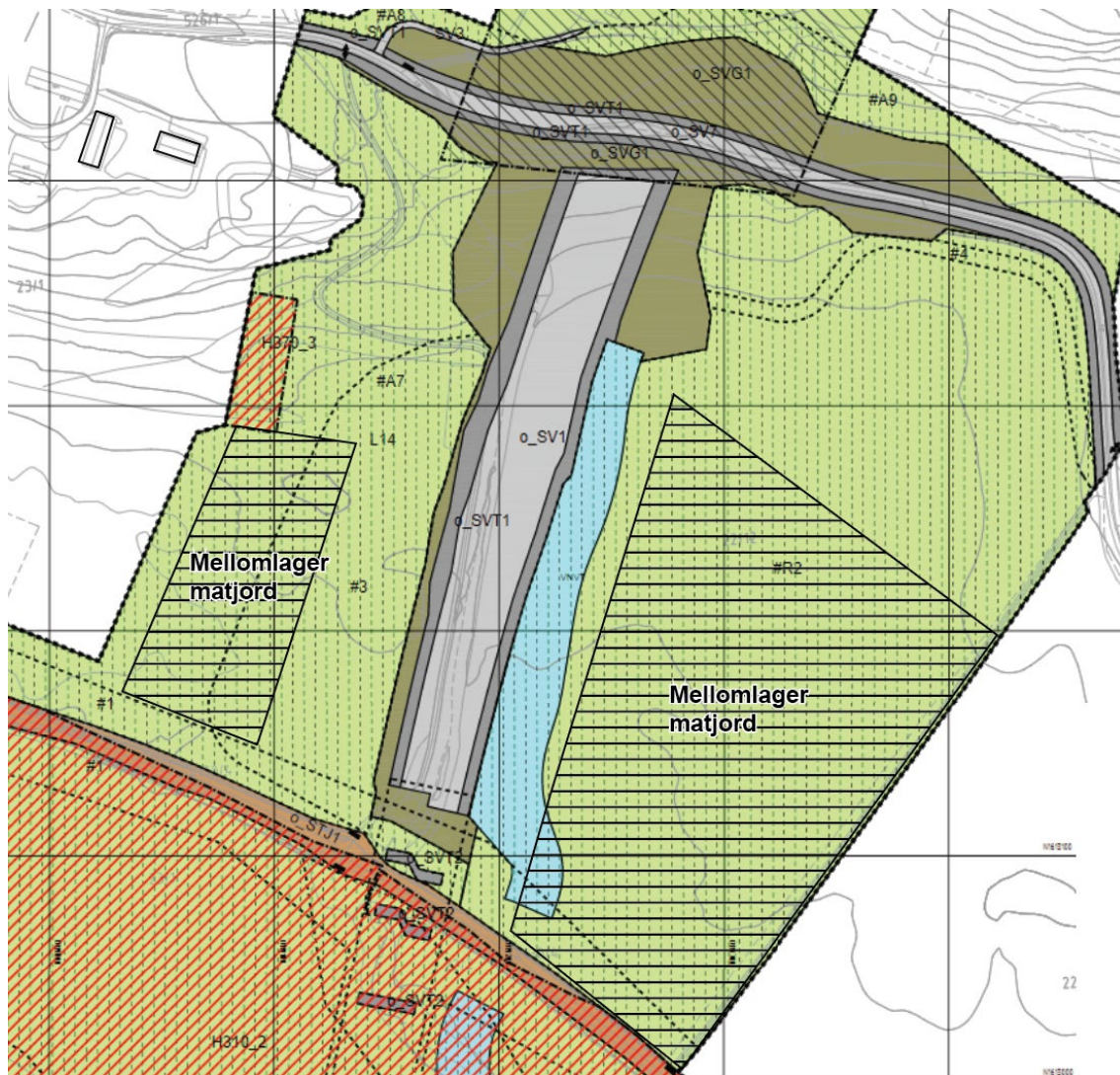
Figur 20 Berørte områder for veianlegget ved Holan med inntegnet vei (permanent beslag) og områder som skal tilbakeføres til jordbruksareal vest og øst for veilinen. Det er skissemessig angitt areal for midlertidig lagring av jordmasser.
