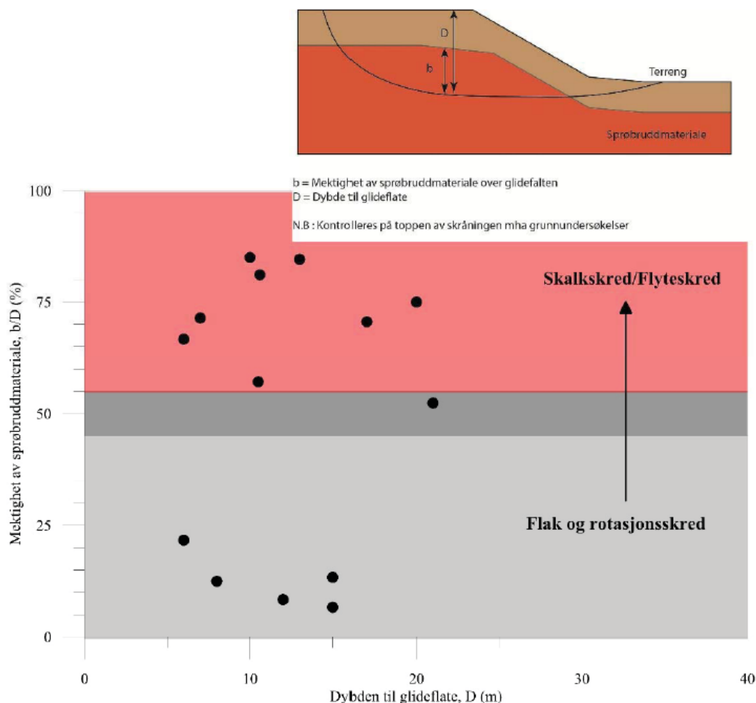
Figur 6 Prinsipp for vurdering av skredmekanisme, hentet fra NIFS-rapport 14/2016 [2].
