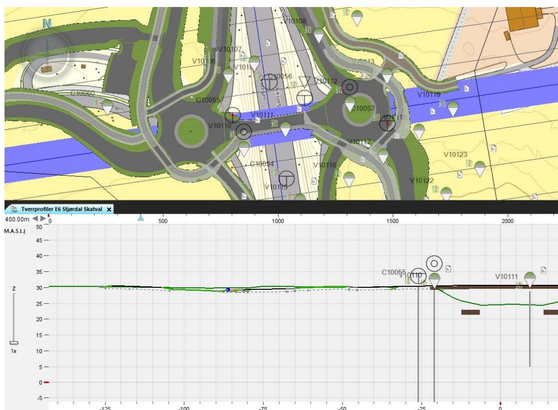
Figur 17 Plan og profil gjennom Kvithammarkrysset.
