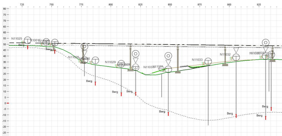
Figur 30 Lengdesnitt av Vollselvbrua akse 1-6.
