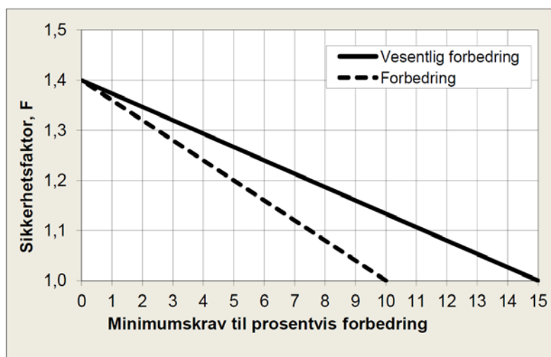
Figur 5 Prinsipp for krav til prosentvis forbedring av sikkerhet.
