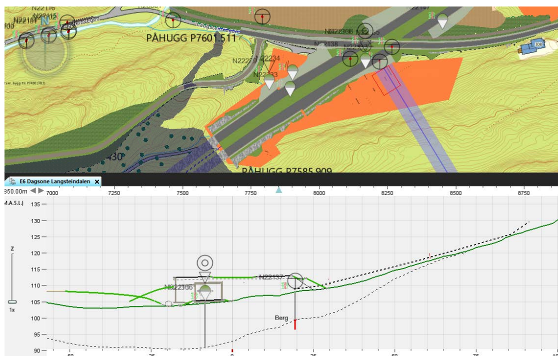
Figur 26 Plan og profil av riggområde (oransje) nord for Forbordsfjelltunnelen.
