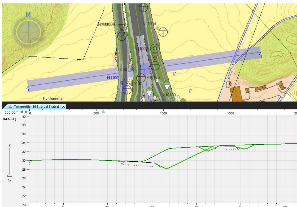
Figur 21 Plan og profil av nordgående påkjøringsrampe fra Kvithammarkrysset. Skjæringen er ca. 4,5 m dyp og med adkomstveg oppå.
