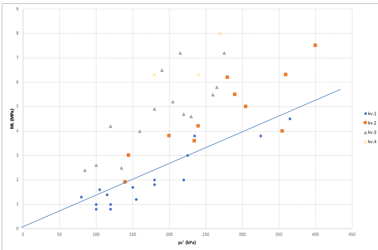
Figur 15 Sammenstilling av M_L mot p_c' og valgt trendlinje for alle tolkede ødometerforsøk i området. De ulike symbolene angir prøvekvalitet, der kvalitet 1 er best og kvalitet 4 er dårligst.
