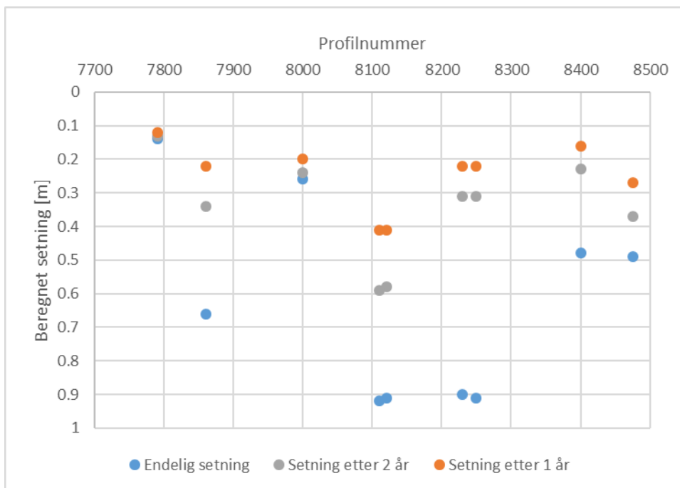
Figur 18 Beregnede totale setninger og setninger etter 1 og 2 år, forutsatt full fyllingshøyde ved tid null.
