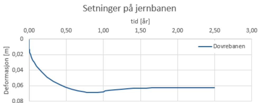
Figur 17 Beregnede deformasjoner på Nordlandsbanen.
