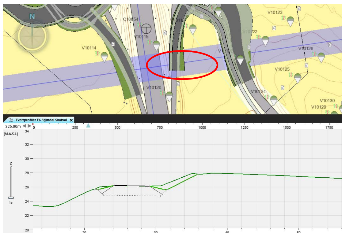
Figur 19 Plan og profil av nordgående avkjøringsrampe til Kvithammarkrysset, kun små terreng-inngrep, mindre enn 2 m dybde.
