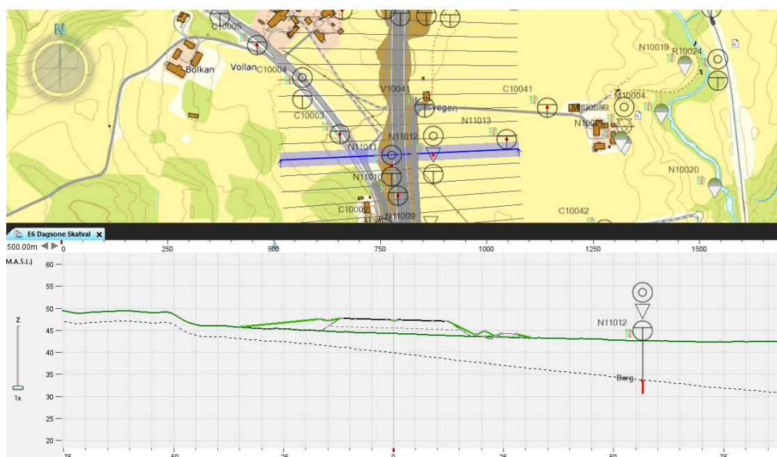
Figur 5 Plan og profil ca. 500 m nord for Kvithammarkrysset. E6 ligger her på 3,2 m fylling og berget synker østover.
