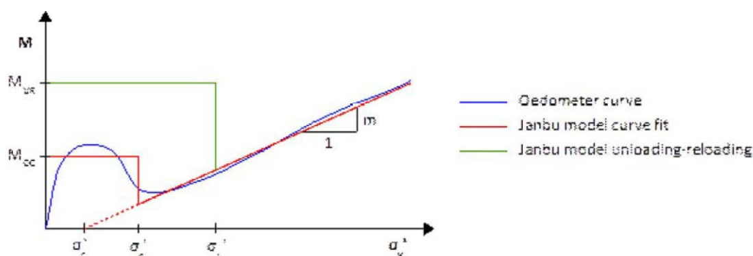
Figur 11 Prinsipp for beregning av setninger etter Janbu, hentet fra Geosuites brukermanual.
