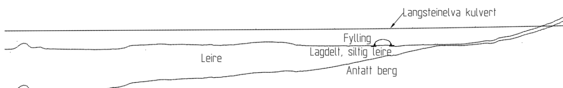
Figur 7 Lengdesnitt gjennom vegfylling i nordligste del av Langsteindalen. Ca. profil 8230-8590.
