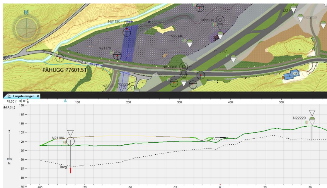
Figur 22 Plan og profil av Langsteinvegen vest for Langsteinvegen undergang.
