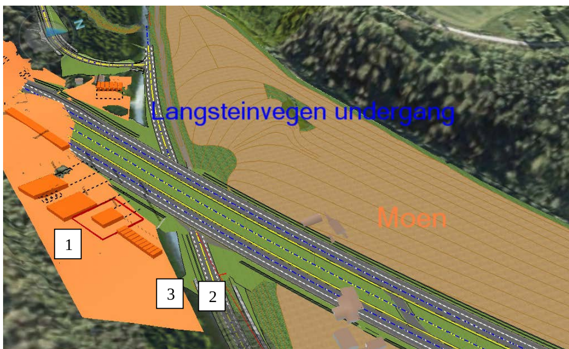
Figur 16 Sør for kulverten for Langsteinvegen skal det etableres et riggområde, vist med oransje (1). Etablering av kulvert og riggområde medfører både skjæring i eksisterende terreng (2) og fylling på toppen (3).
