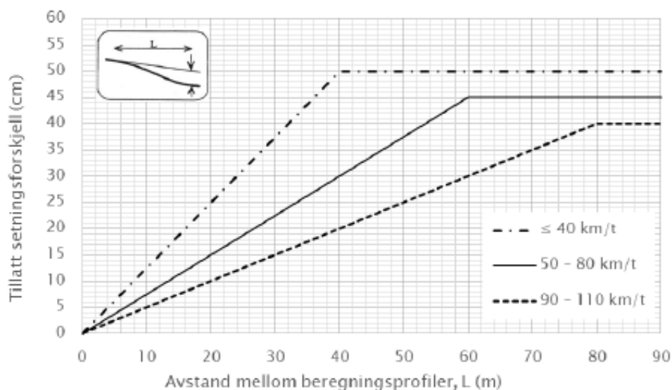
Figur 10 Krav til setninger for veglinje, hentet fra N200 [1].
