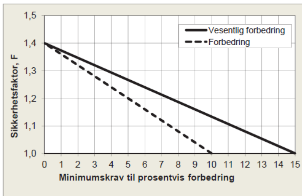
Figur 7 Krav til prosentvis forbedring ved topografiske endringer eller bruk av lette masser. [6]
