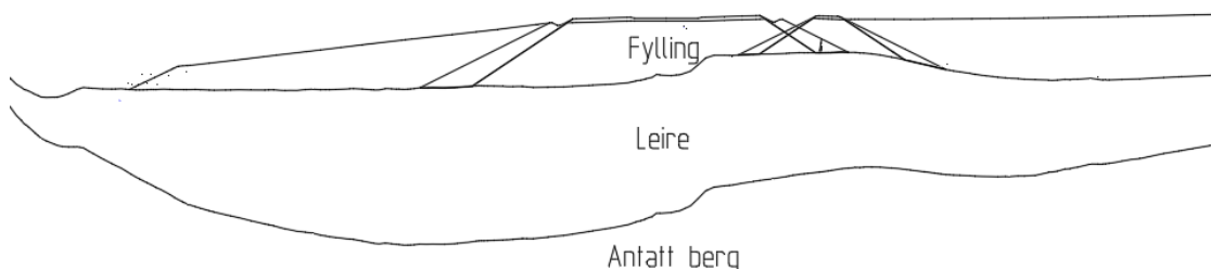
Figur 9 Tverrsnitt gjennom vegfylling i profil 8250. Relativt høy fylling i nordligste halvdel av Langsteindalen.
