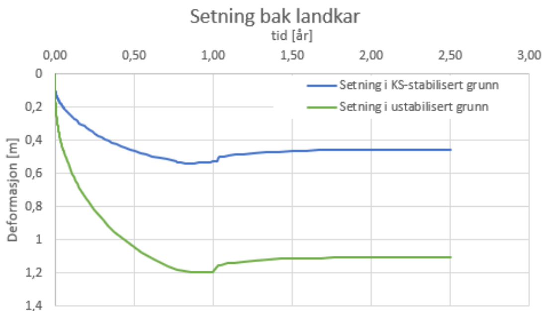
Figur 16 Beregnede setninger bak landkar. Beregninger utført for leire med og uten grunnforsterkning.
