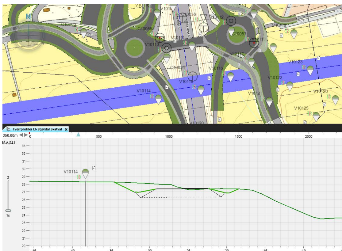
Figur 16 Plan og profil av sørgående på-rampe.
