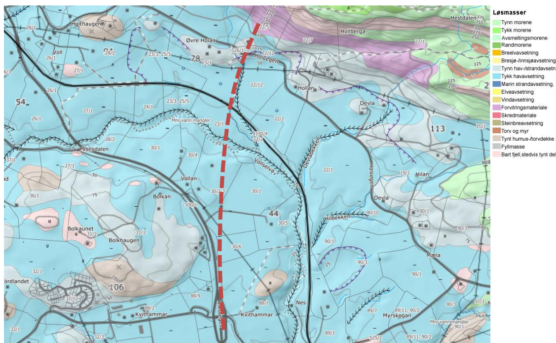
Figur 3 Kvartærgeologisk kart over området. Omtrentlig plassering av veglinja er vist med rød stiplert linje.
