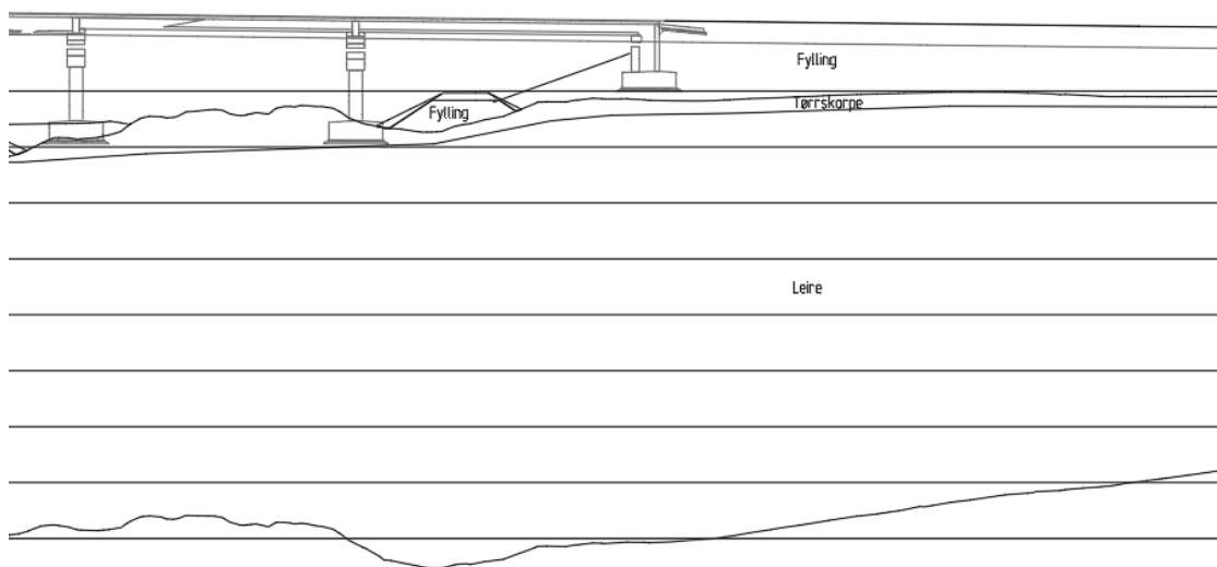
Figur 3 Lengdesnitt av fyllinga ved Nordlandsbanen. Dybden til berg ved landkaret er ca. 40 meter, og avtar gradvis bakover mot tunnelpåhugget. Avstand mellom de horisontale linjene er 5 meter.
