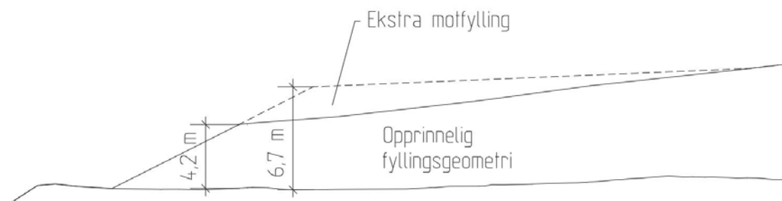
Figur 11 Prinsipp for geometriendring for fyllingen i Langsteindalen.
