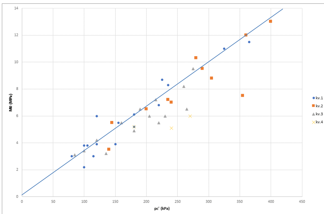
Figur 14 Sammenstilling av M_0 mot p_c' og valgt trendlinje for alle tolkede ødometerforsøk i området. De ulike symbolene angir prøve kvalitet.
