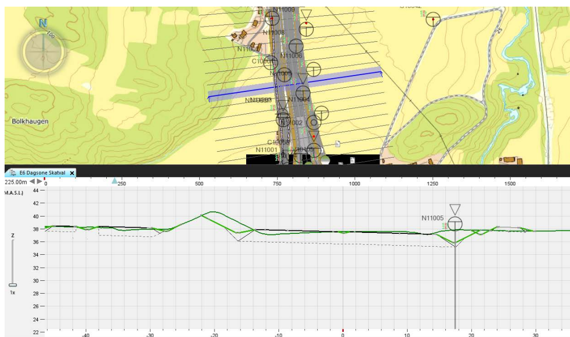
Figur 4 Plan og profil ca. 250 m nord for Kvithammarkrysset. Vegen ligger nøytralt i terrenget, men det blir mindre skjæringer for nye grøfter.
