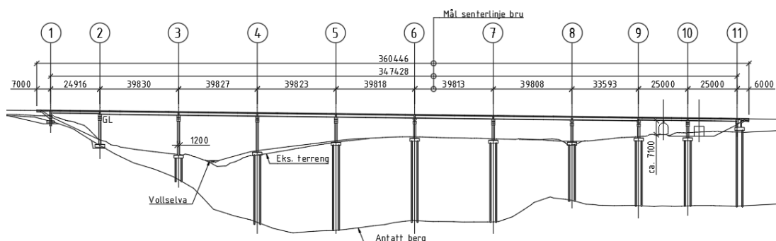
Figur 37 Oppriss av nordgående Vollselvbru.
