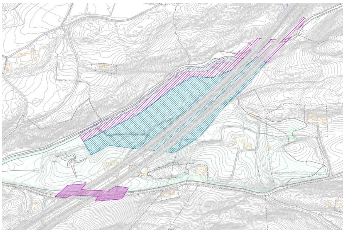
Figur 13 Fyllingen i Langsteindalen. Estimert areal som må forsterkes med kalksement er vist med lilla skravur, mens område det må installeres vertikaldren er vist med blå skravur. Gjengitt på tegning 015.
