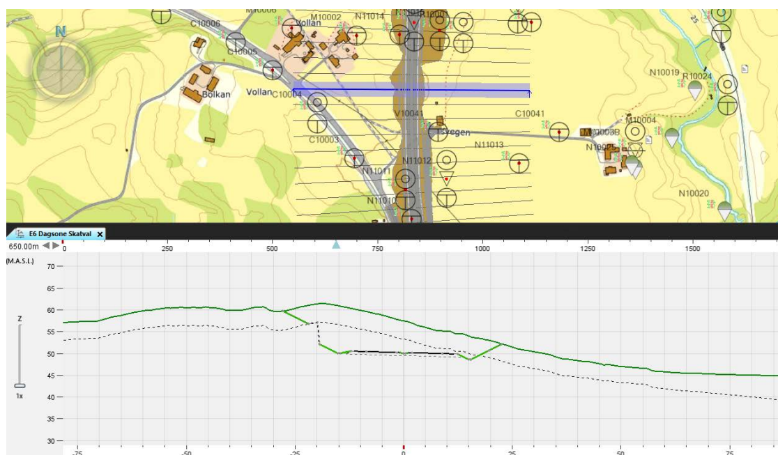
Figur 6 Plan og profil ca. 650 m nord for Kvithammarkrysset. Ca. 11,5 m skjæring gjennom en terrengrygg med liten løsmasseoverdekning.
