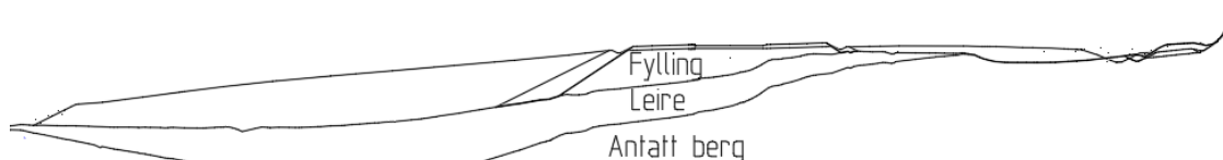
Figur 8 Tverrsnitt gjennom vegfylling i profil 8000. Relativt lav fylling i sørligste halvdel av Langsteindalen. Løsmassemekktigheten øker mot vest.
