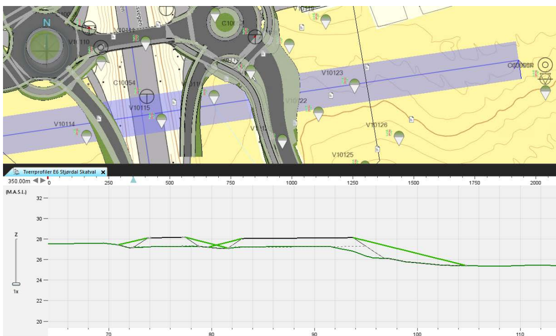
Figur 20 Plan og profil av William Holmens veg sørøst for Kvithammarkrysset. Vegen legges ut på en inntil 2 m høy fylling inn mot rundkjøringen.
