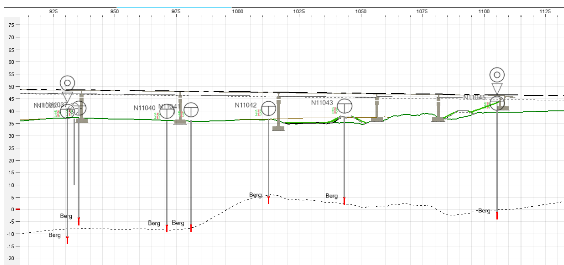
Figur 31 Lengdesnitt av Vollselvbrua akse 6-11.
