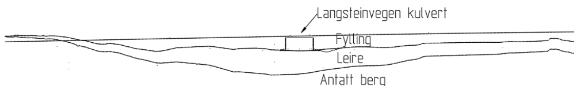
Figur 5 Lengdesnitt gjennom vegfylling i sørligste del av Langsteindalen. Ca. profil 7730-8000.
