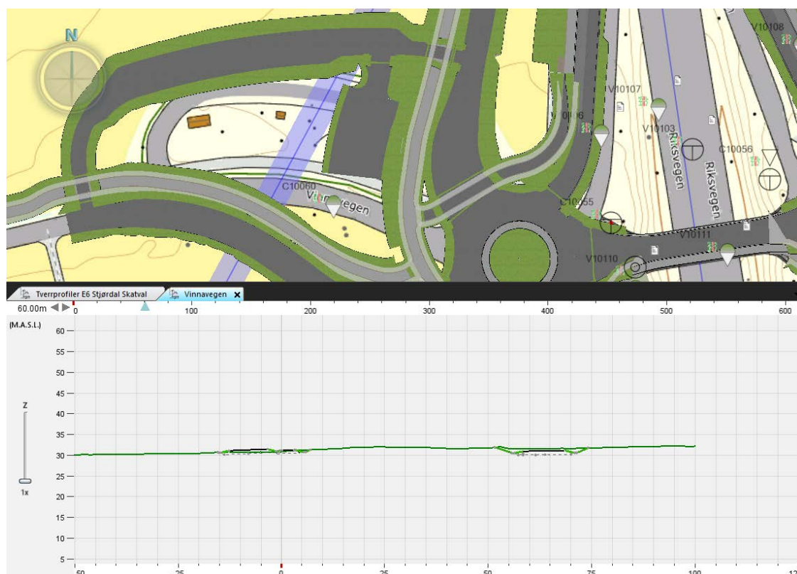
Figur 15 Plan og profil av rasteplassen på Kvithammar, terrengendringer er mindre enn 1 m.
