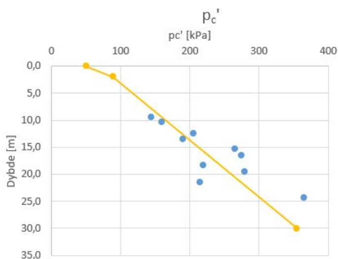
Figur 12 Sammenstilling av prekonsolideringsspenning, p_c' , mot dybden for ødometerforsøk fra borhull N11045 og N11036 ved fyllingen.
