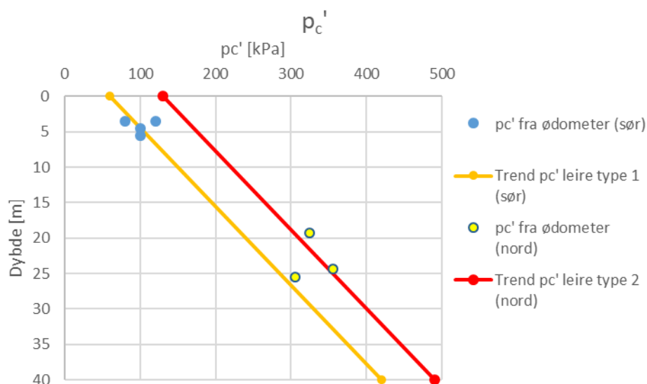
Figur 13 Sammenstilling av prekonsolideringsspenning, p_c' , mot dybden for ødometerforsøk fra borhull N22133 (sør), N22136 (sør) og N22109 (nord) ved fyllingen i Langsteindalen, samt trendlinjer for p_c' i sørlig og nordlig del av Langsteindalen.
