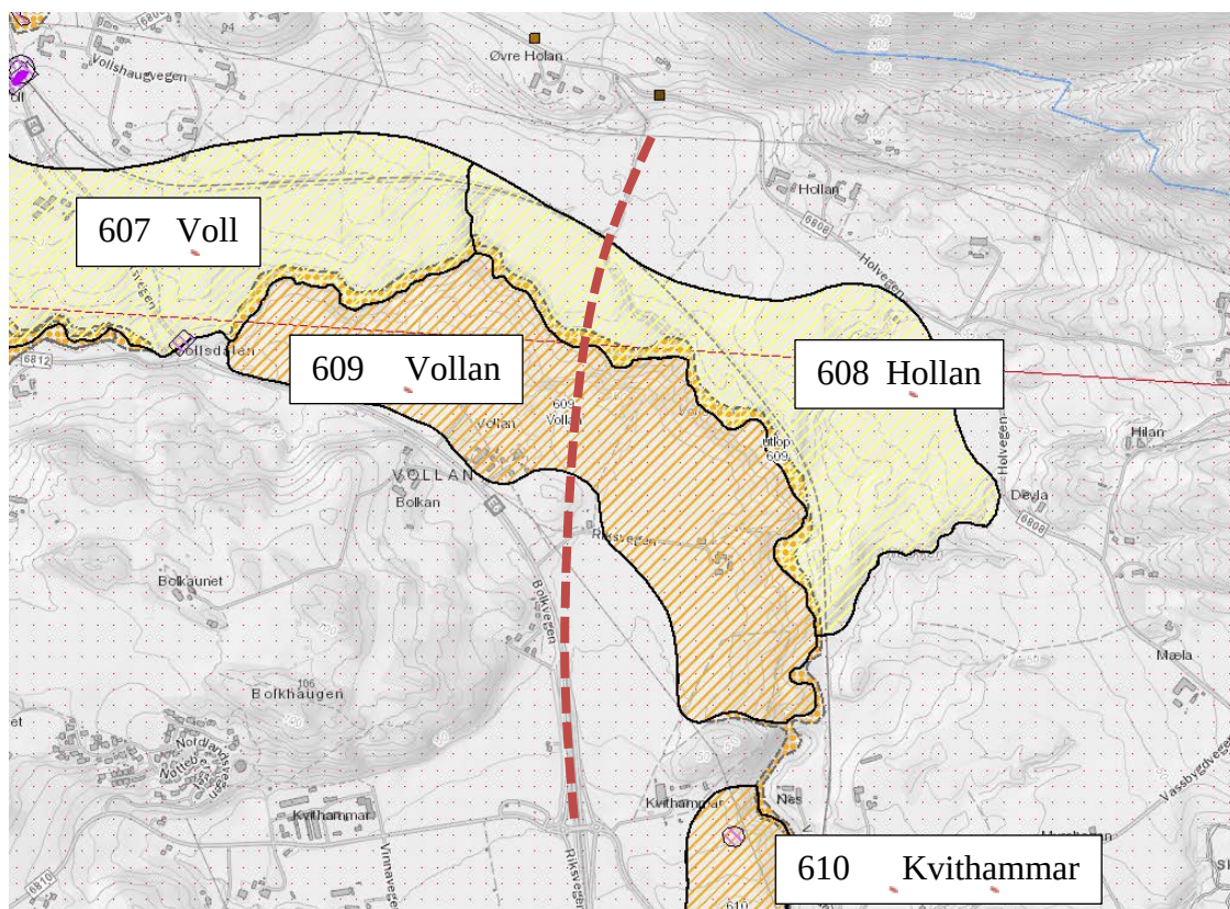
Figur 3 Kartlagte kvikkleirefaresoner. Ny E6 er skissert med rødt. [2]
