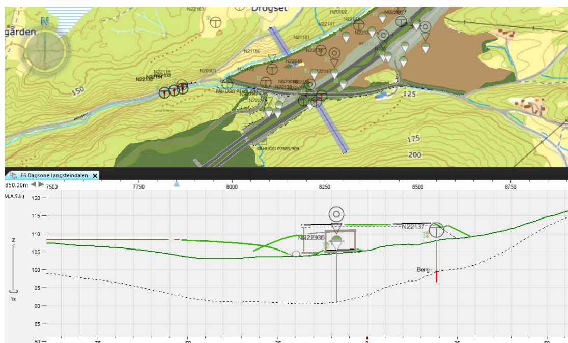
Figur 33 Plan og profil ved Langsteinvegen undergang.
