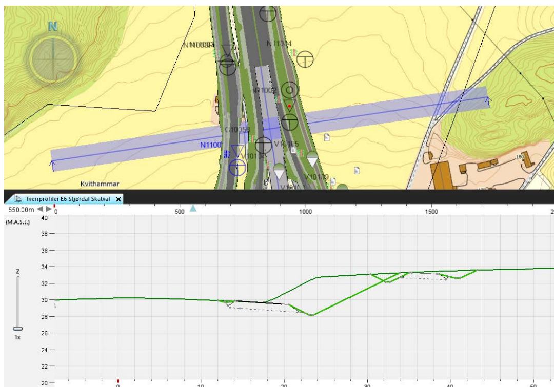
Figur 15 Skjæring ved Kvithammarkrysset. Skjæringen er ca. 4,7 meter høy og med en adkomstveg oppå.
