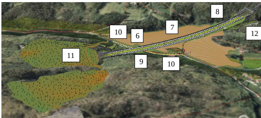
Figur 2 Oversikt over prosjektområdet i Langsteindalen. E6 krysser dalen hovedsakelig på fylling. Dette inkluderer kryssing av Fv.6816 og Langsteinelva. Nede til venstre ses deponier.
