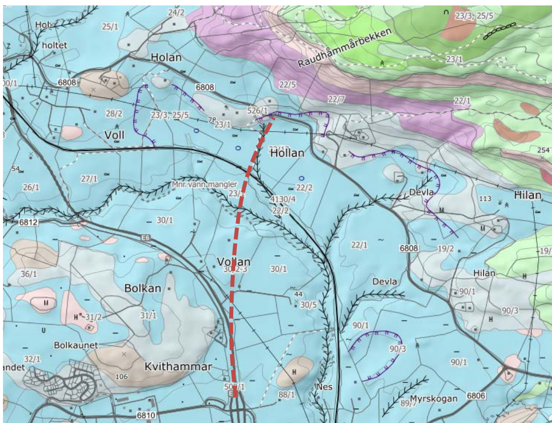
Figur 1 Kvartærgeologisk kart over dagsonen sør for Forbordsfjelltunnelen. E6 traseen er skissert med rød stiplet linje. [1]
